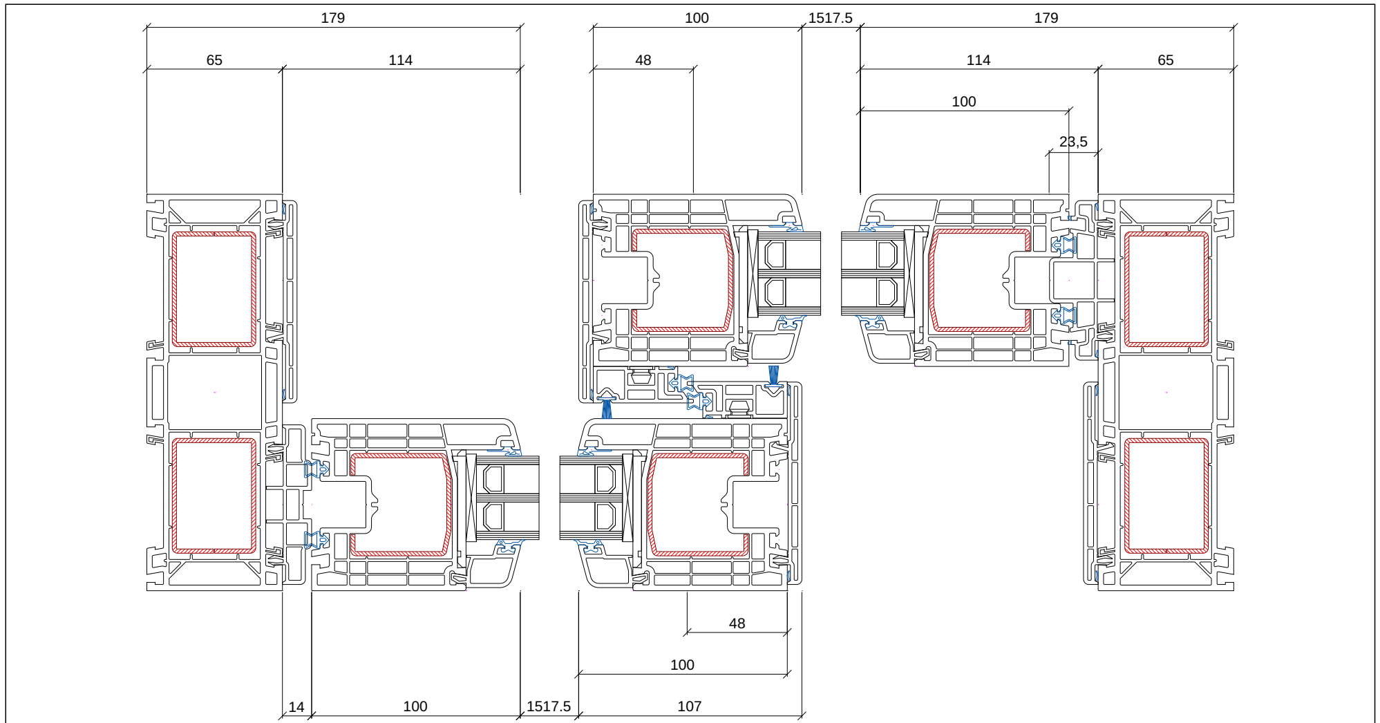
Profil zárubně 6360 Profil zárubně 65 mm Křídlo 6362 Křídlo 100 mm
